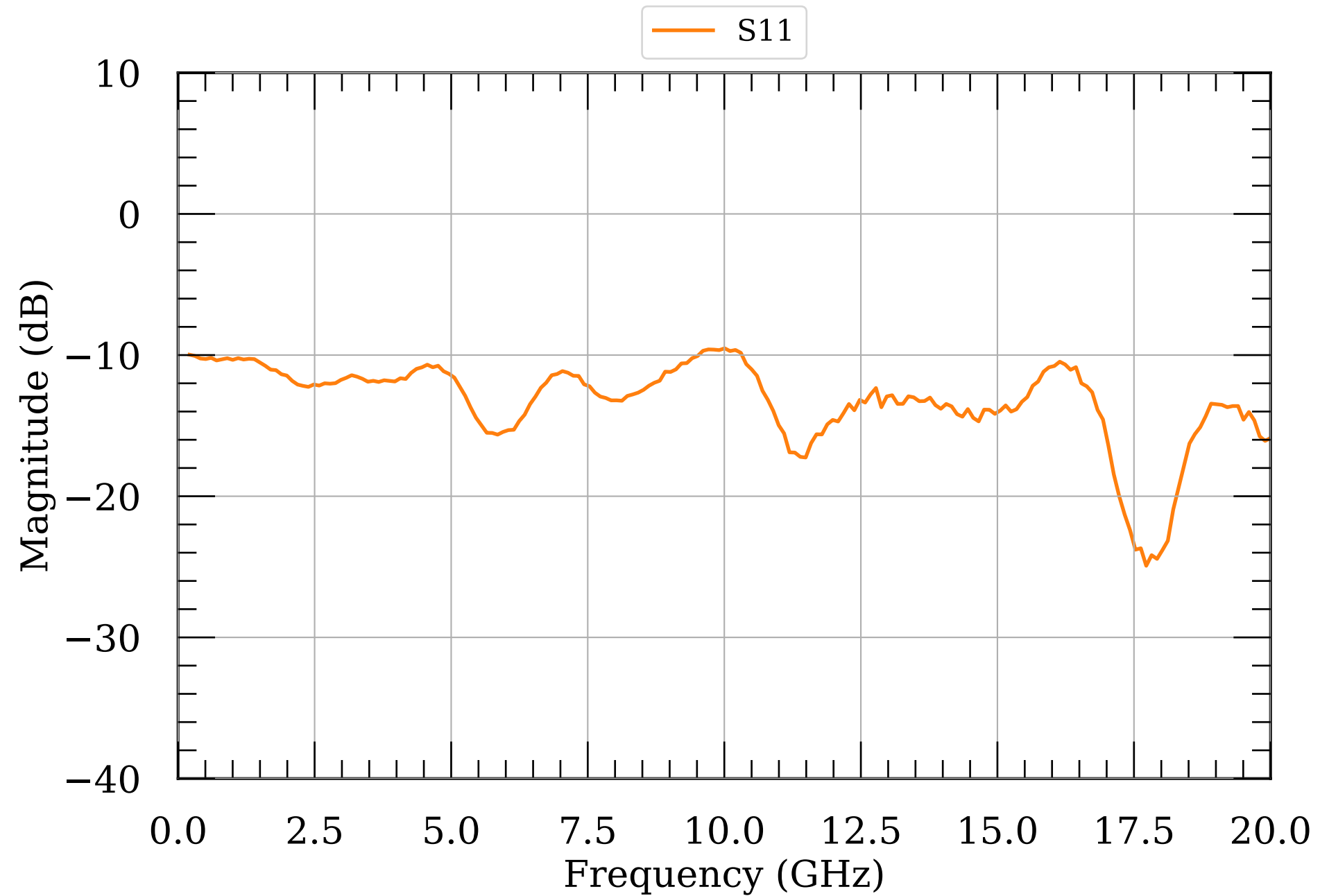
LNA S-params module034v2
